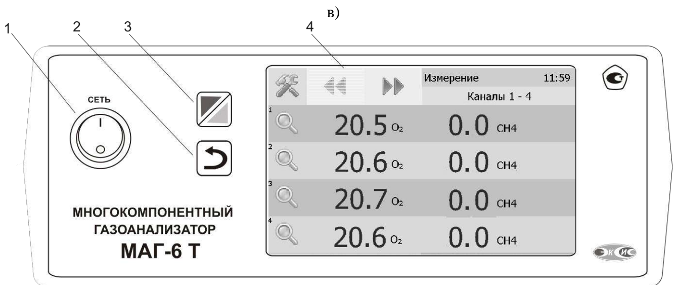
Рисунок 3.1 Вид лицевой панели газоанализатора:
